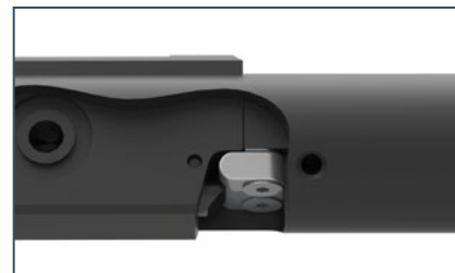
EINSTELLBARE LAUFAUSRICHTUNG MIT VERBES- SERTEM VERRIEGELUNGSMECHANISMUS ADJUSTABLE BARREL ALIGNMENT WITH IMPROVED LOCKING MECHANISM
